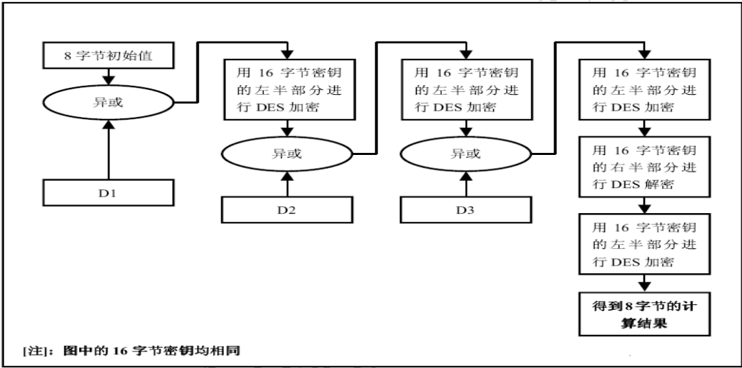
图 3.18 用Triple DES密钥产生MAC的算法
