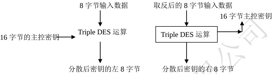
图 3-10 Triple DES 密钥分散
