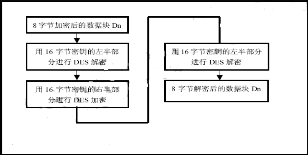
图 3.22 用Triple DES密钥进行数据解密计算
